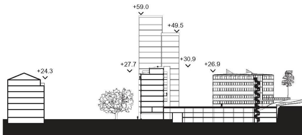
Sektion genom Gustavslundsvägen och Racketen 11 med det tvådelade höghuset, låghuset med indragen takvåning och parkeringsgaraget i tre plan. Till vänster befintliga kontor norr om vägen och till höger befintliga kontor i Racketen 10.
