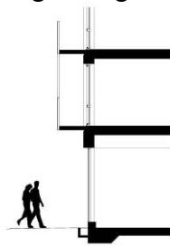
Smala låghusbalkonger mot torgytan Olika djupa balkonger ger varierad fasad
